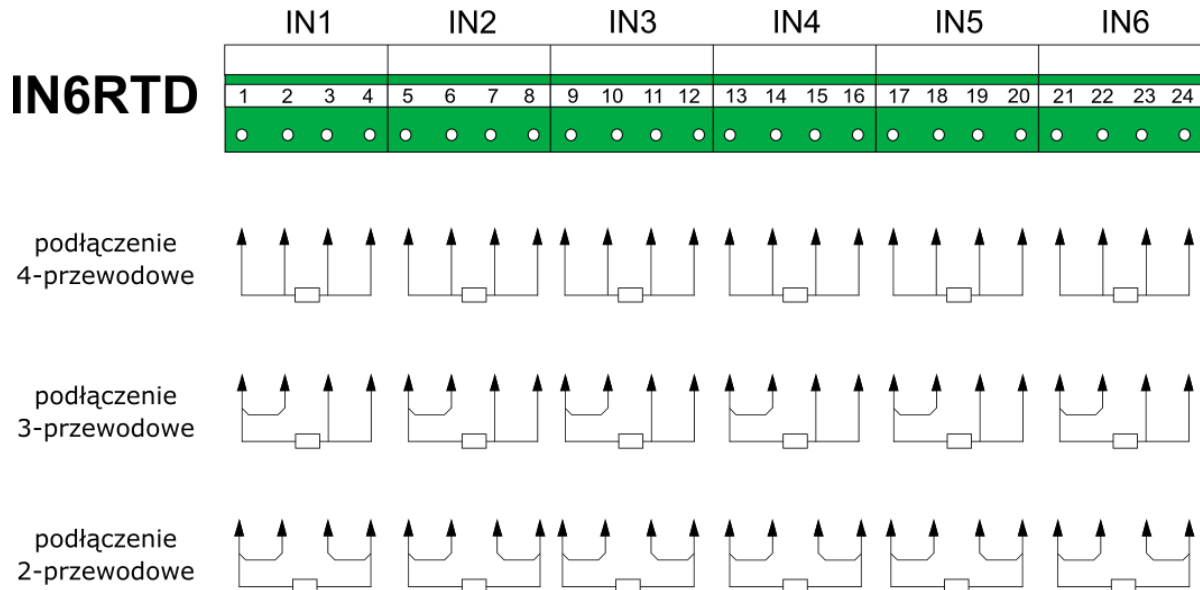
Rys. 6.5 Schemat połączeń dla modułu IN6RTD.
