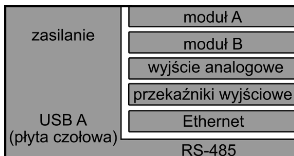
Rys. 3.1 Separacja galwaniczna w DL2 (separacja funkcjonalna 500VAC @ 1min).
