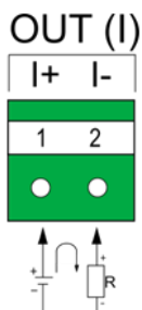
Rys. 6.22 Schemat podłączenia wyjścia analogowego.
