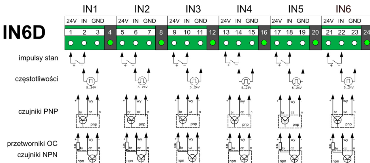
Rys. 6.22 Schemat podłączeń dla modułu IN6D.
