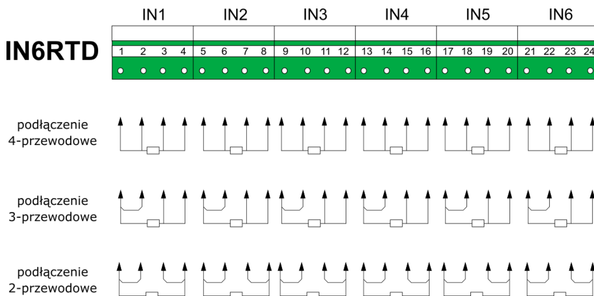
Rys. 6.5 Schemat podłączeń dla modułu IN6RTD.
