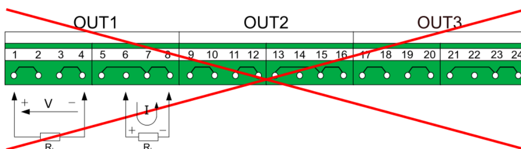
Rys. 6.19 Niepoprawne podłączenie dla modułu OUT3.
