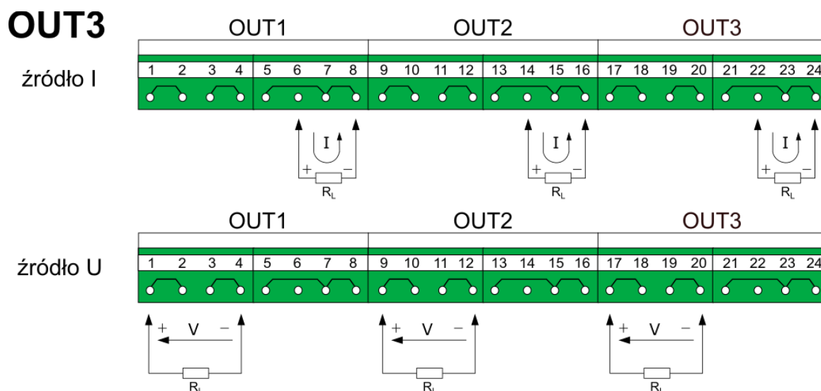
Rys. 6.17 Schemat połączeń dla modułu OUT3.
