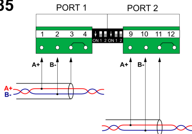
Rys. 6.14 Schemat podłączeń dla modułu 2RS485.
