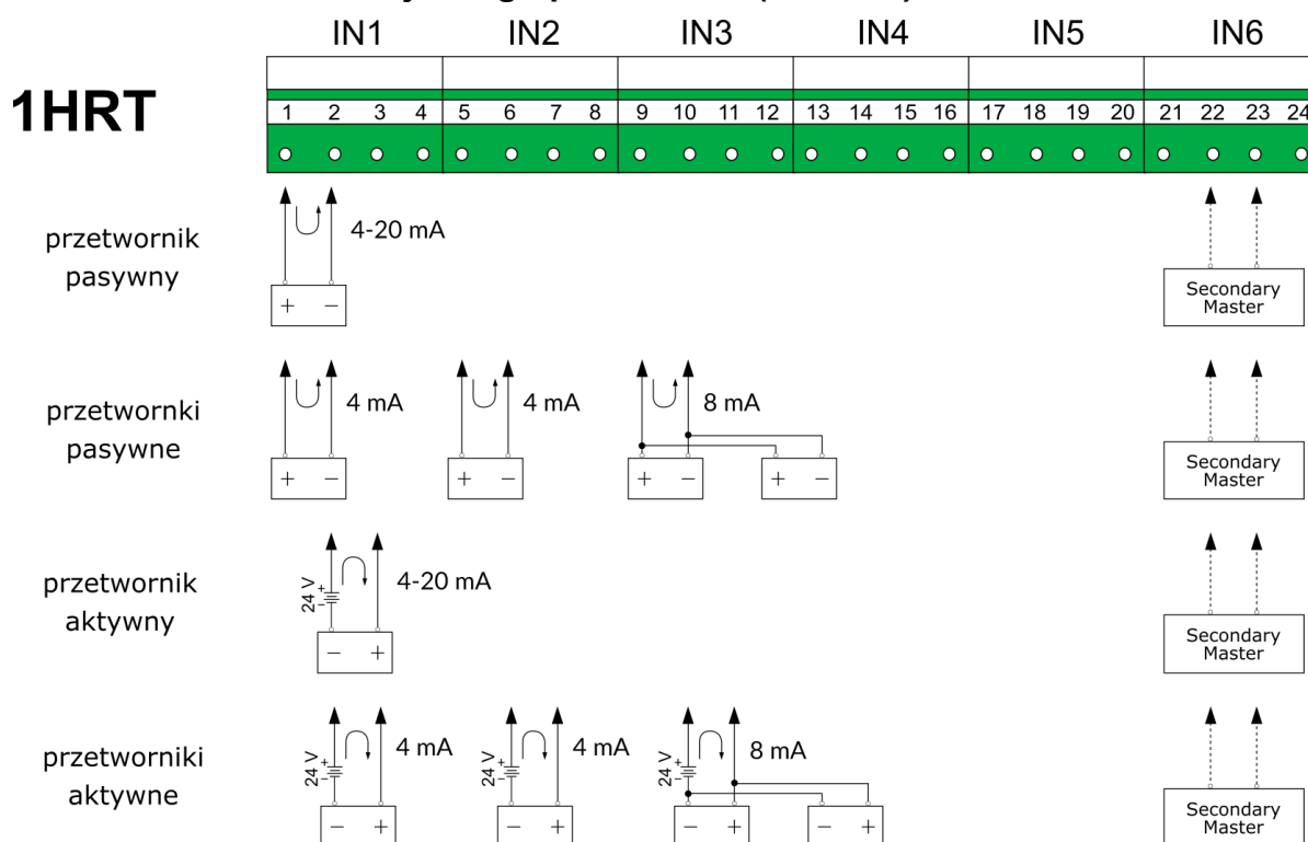
Rys. 6.15 Schemat połączeń dla modułu 1HRT.
