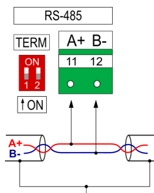
Rys. 6.24 Schemat podłączenia RS-485.
