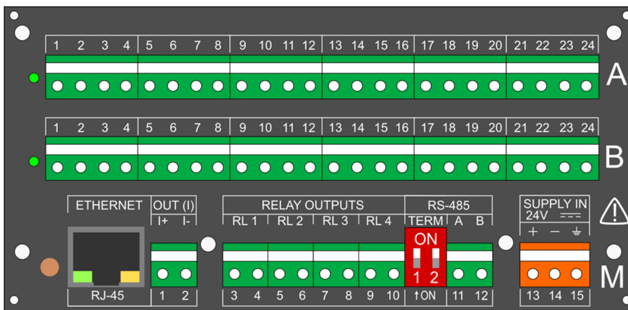
Rys. 6.1 Przykładowy widok płyty tylnej DL2.
