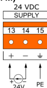
Rys. 6.2 Schemat podłączenia zasilania.
