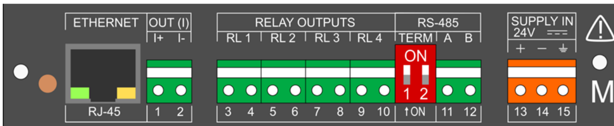
Rys. 6.21 Widok płyty tylnej urządzenia (Moduł M).
