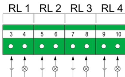
Rys. 6.23 Schemat podłączenia wyjść przekaźnikowych.
