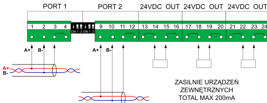
Rys. 6.13 Schemat połączeń dla modułu 2RS485(24V).
