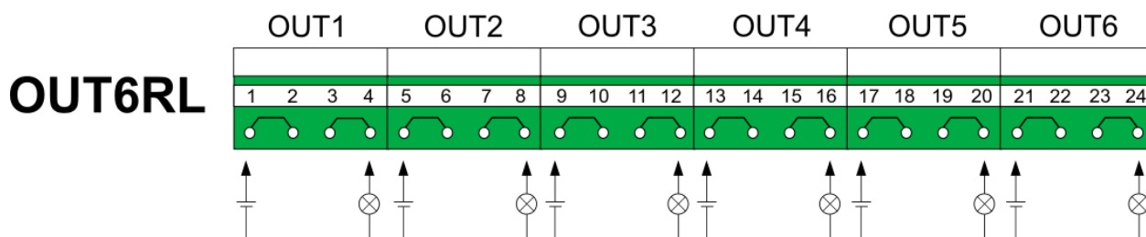
Rys. 6.16 Schemat połączeń dla modułu OUT6RL.
