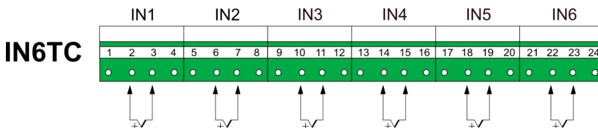
Rys. 6.7 Schemat podłączeń dla modułu IN6TC.
