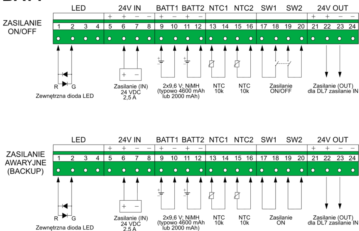
Rys. 6.20 Schemat podłączeń dla modułu PSBATT.
