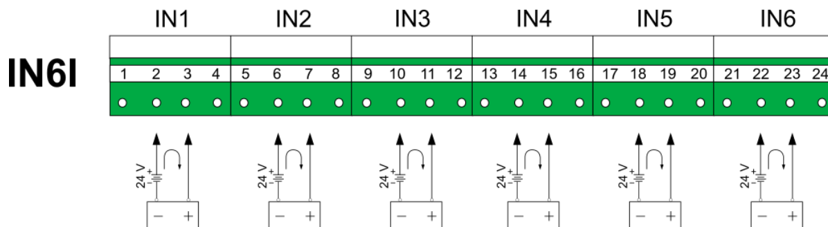
Rys. 6.4 Schemat podłączeń dla modułu IN6I.
