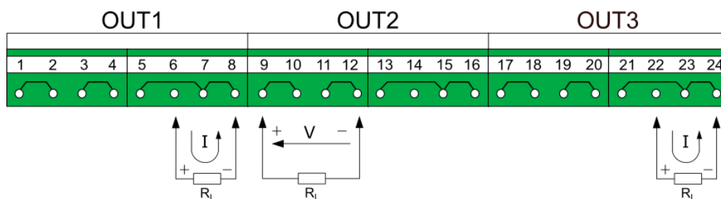
Rys. 6.18 Poprawne podłączenie dla modułu OUT3.
